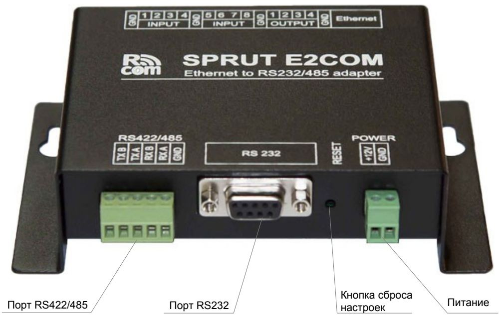
Рис. 2.4 Вид сзади
